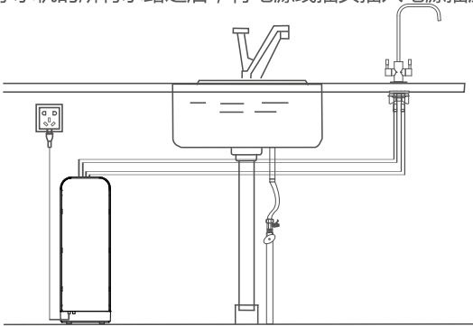
电路安装示意图
